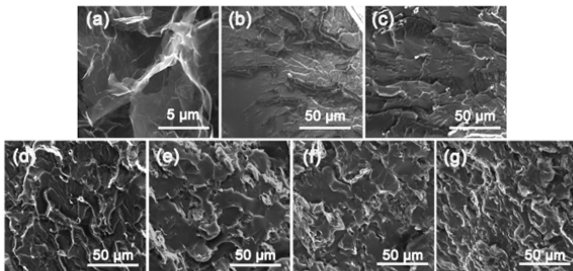
شکل ۱: تصاویر SEM از (a) MLG استفاده شده و سطح شکست فیلم های کامپوزیت MLG/PVC حاوی مقادیر مختلف از MLG (b) ۰، (c) ۰/۵، (d) ۱/۰، (e) ۲/۵، (f) ۳/۵، (g) ۴/۵ wt%.
